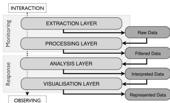
Figura 1: Modelo de capas de COLMENA
