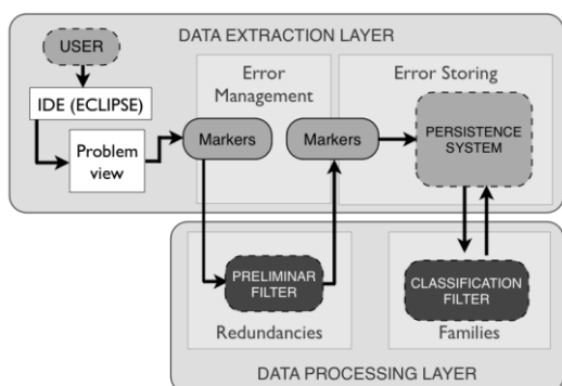
Figura 3: Operaciones de las capas de extracción y procesado
